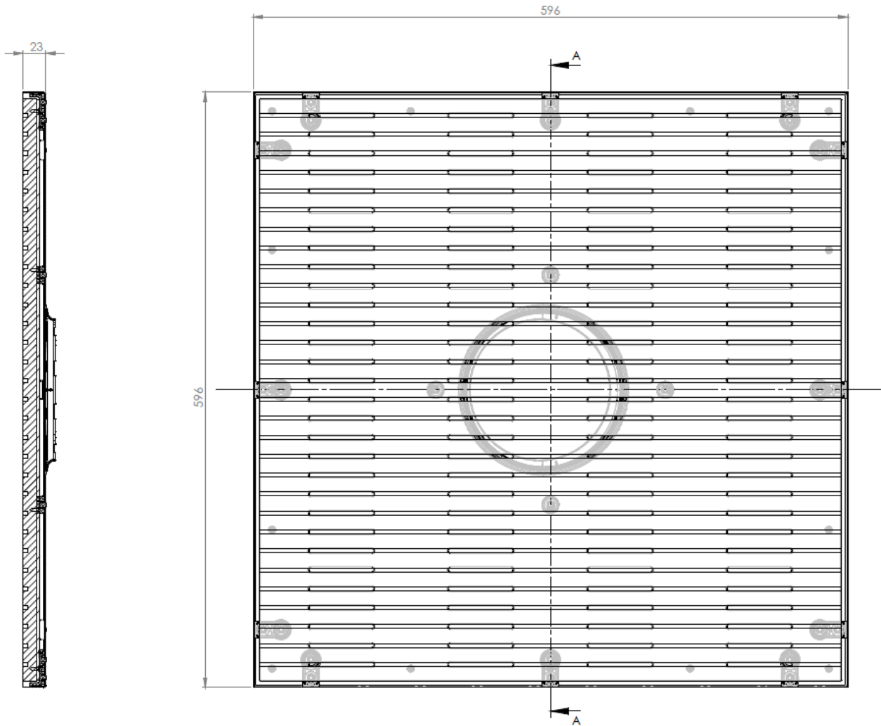
SECTION A-A SCALE 1 : 3
